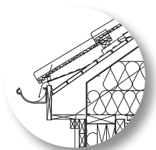
Princip för utförande med kort takfot.
